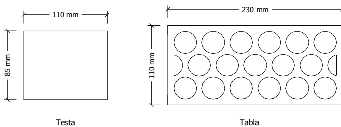
Croquis de la pieza. Cotas en mm
