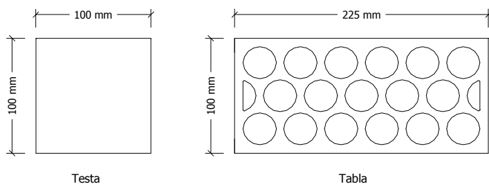
Croquis de la pieza. Cotas en mm
